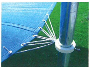
Abdeckung und Sonnenschutz mit ø 89mm Pfosten und Polyamid-Stellung
